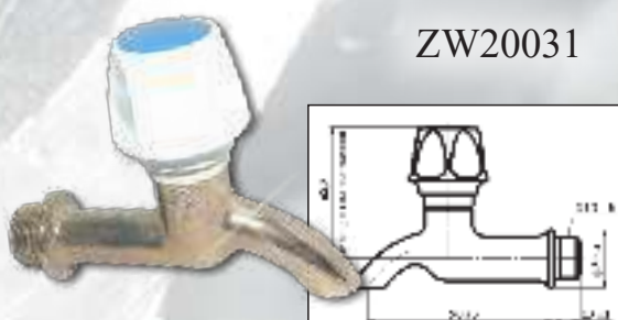
Кран водоразборный настенный
